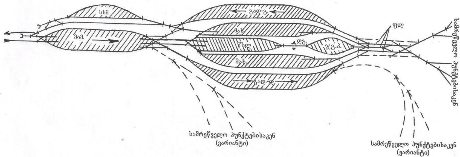
ნახ. 1 რკინიგზის სამრეწველო მახარისხებელი სადგურის სქემა დიდი მოცულობით გაგონნაკადის გადამუშავების პირობებში
